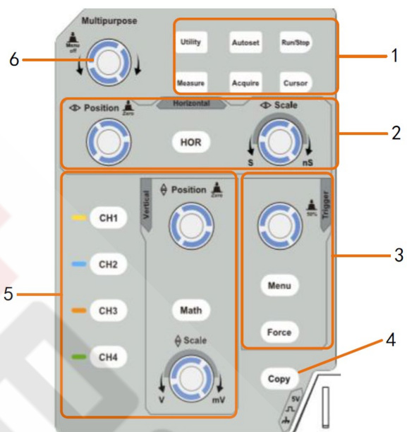
Рисунок 3.3. Общий вид панели управления
