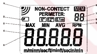
структура ЖК-дисплея
