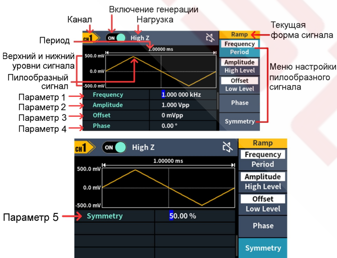
Рисунок 5.5. Интерфейс управления пилообразным сигналом
