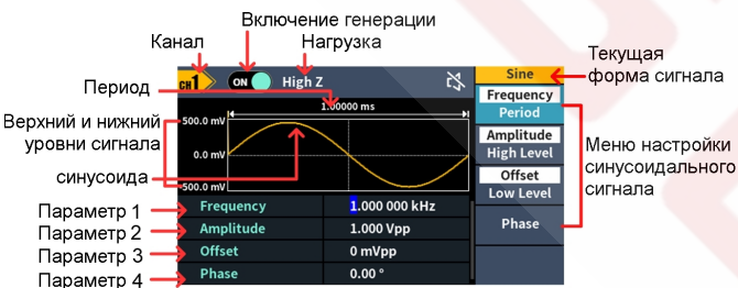
Рисунок 5.2. Интерфейс управления синусоидальным сигналом
