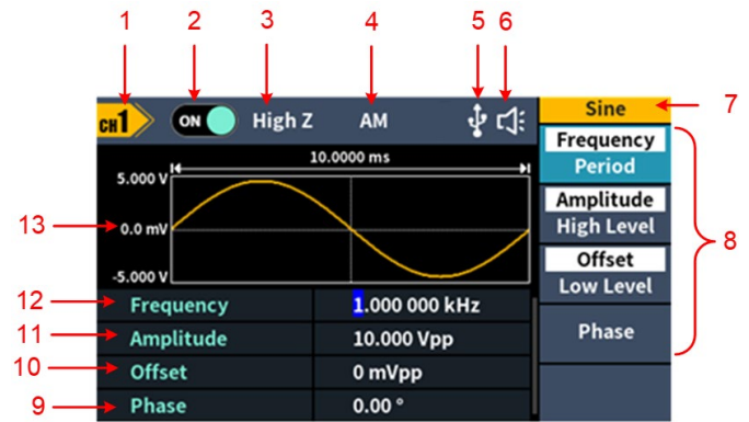
Рисунок 4.3. Интерфейс пользователя
