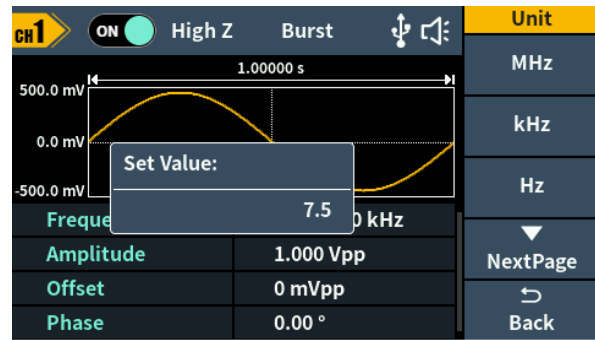
Рисунок 5.3. Использование клавиатуры цифрового ввода для задания частоты
